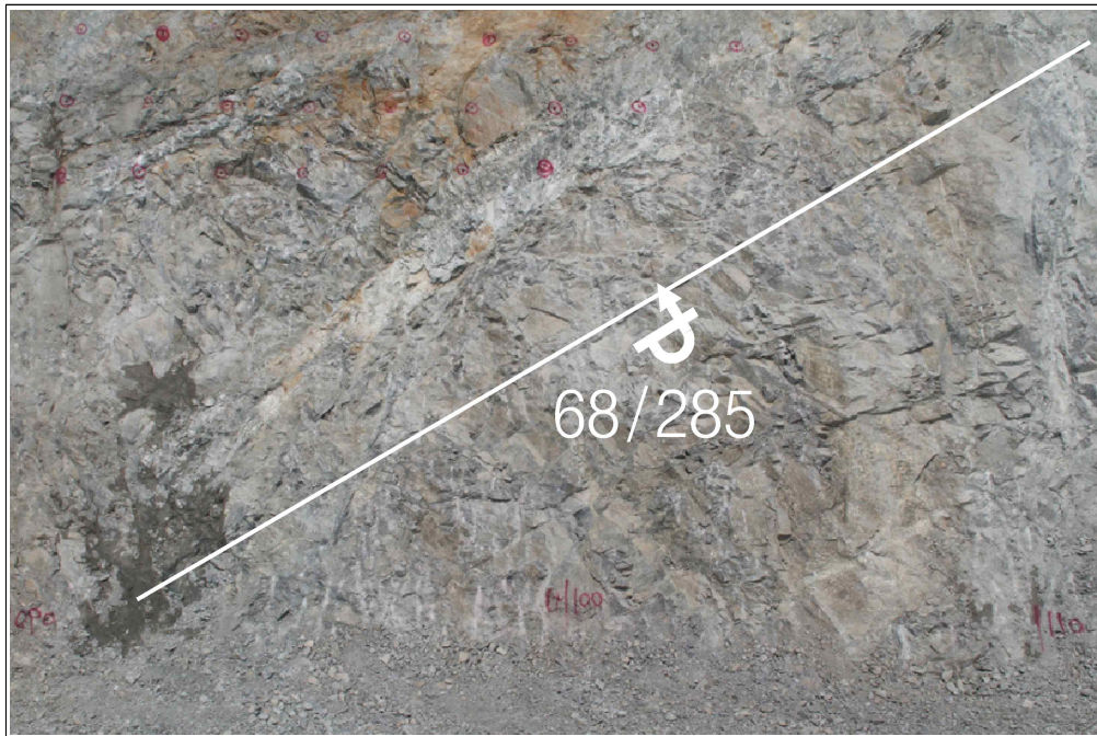
【그림 34】 C 영역에 발달한 불연속면
