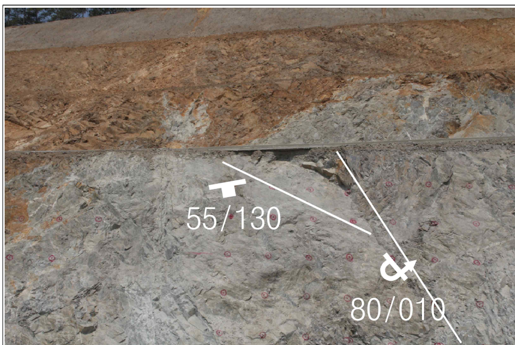
【그림 35】 C 영역에 발달한 불연속면
