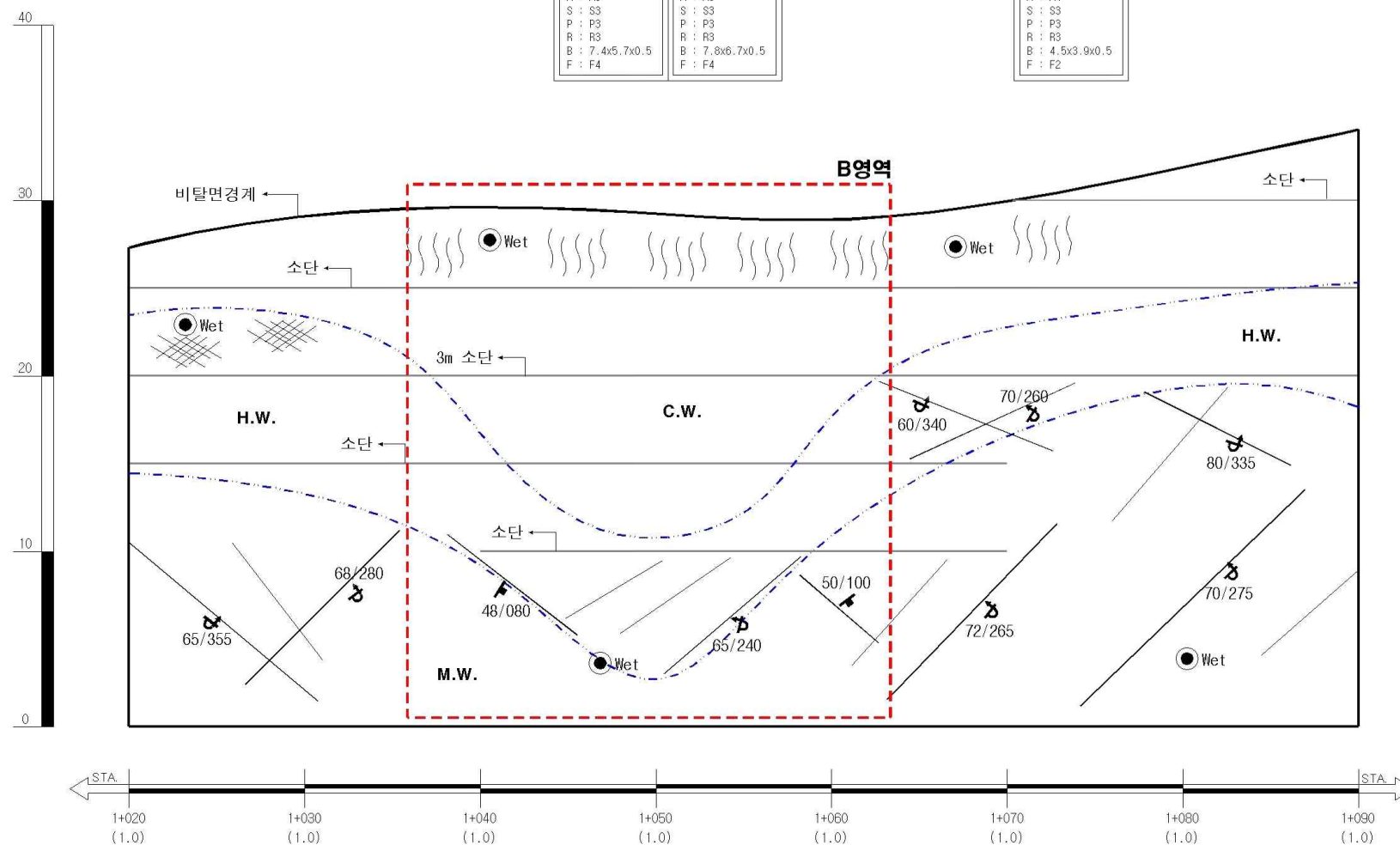
B영역 불연속면 자료
