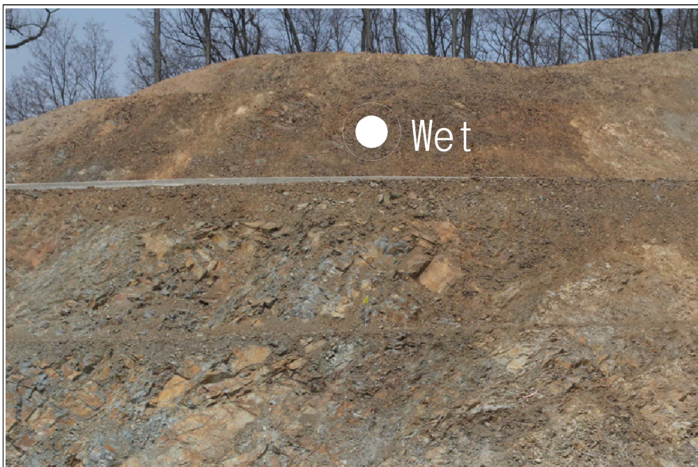
【그림 23】 A 영역 상세사진 (지하수 유출)
