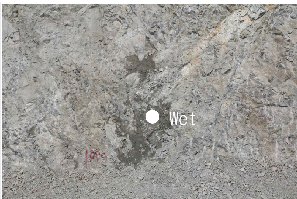
【그림 39】 C 영역 상세사진 (지하수 유출)
