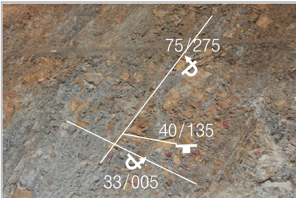
【그림 19】 A 영역에 발달한 불연속면
