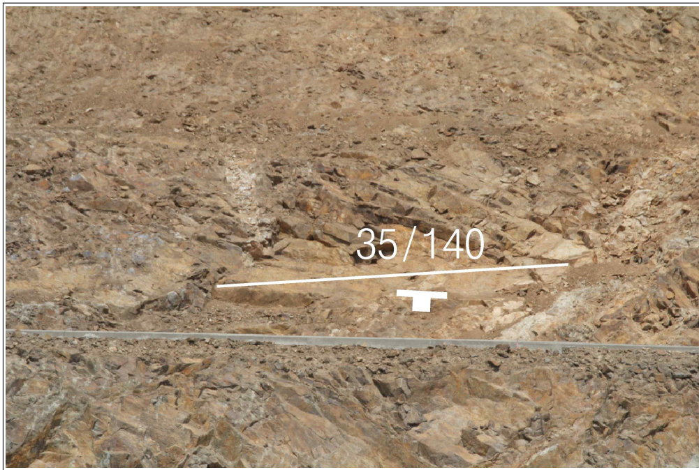
【그림 32】 C 영역에 발달한 불연속면
