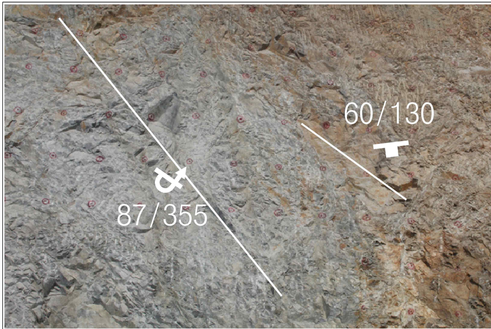
【그림 41】 D 영역에 발달한 불연속면
