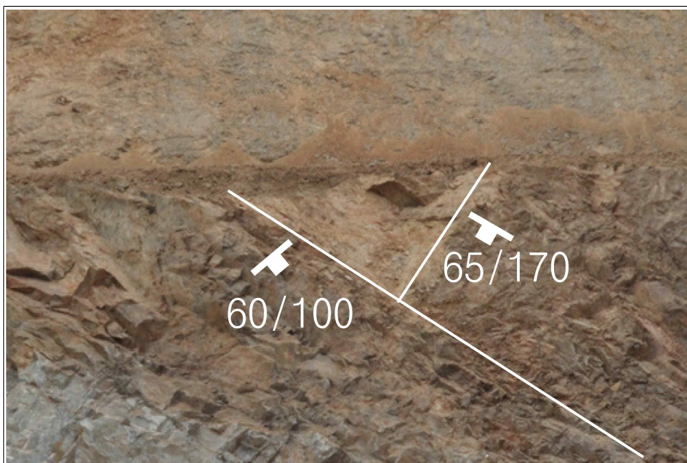
【그림 40】 D 영역에 발달한 불연속면
